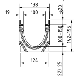
pro NW100 G, Nr. 5-0 f. možný bočný odtok/f. side outlet drilling
