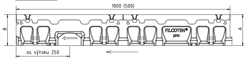
pro NW100 G
