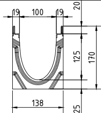
pro NW100 V-E, Nr. 5-0 f. možný bočný odtok/f. side outlet drilling
