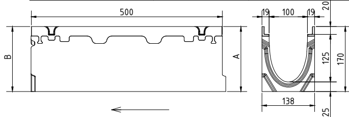
pro NW100 G, Nr. 5-0 f. možný bočný odtok/f. side outlet drilling
