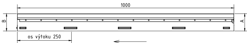
pro NW100 mini 60/80 V-E
