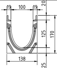
pro NW100 G, Nr. 5-0 f. možný bočný odtok/f. side outlet drilling
