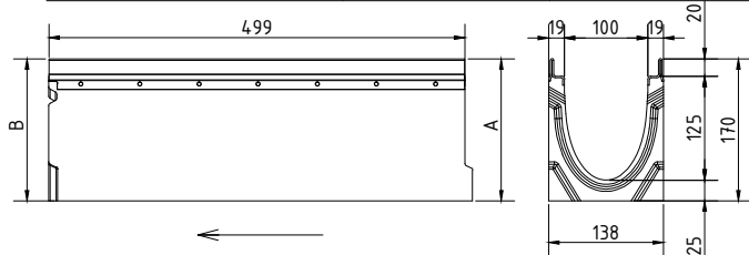
pro NW100 V-E, Nr. 5-0 f. možný bočný odtok/f. side outlet drilling
