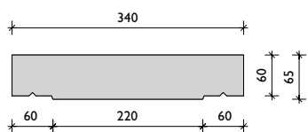
BG KV betónový kryt Gr. 3
