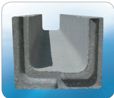
BG-TK 1 Káblový žľab so systémom pero-drážky
